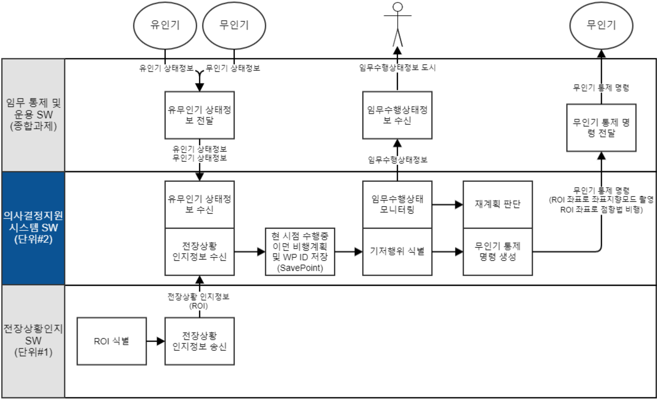
연관 의사결정지원 시스템 내부 운용흐름도
